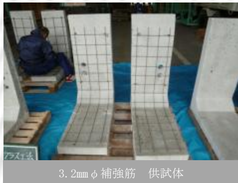
3.2mm φ ・ 6.0 φ mm 補強筋 供試体
